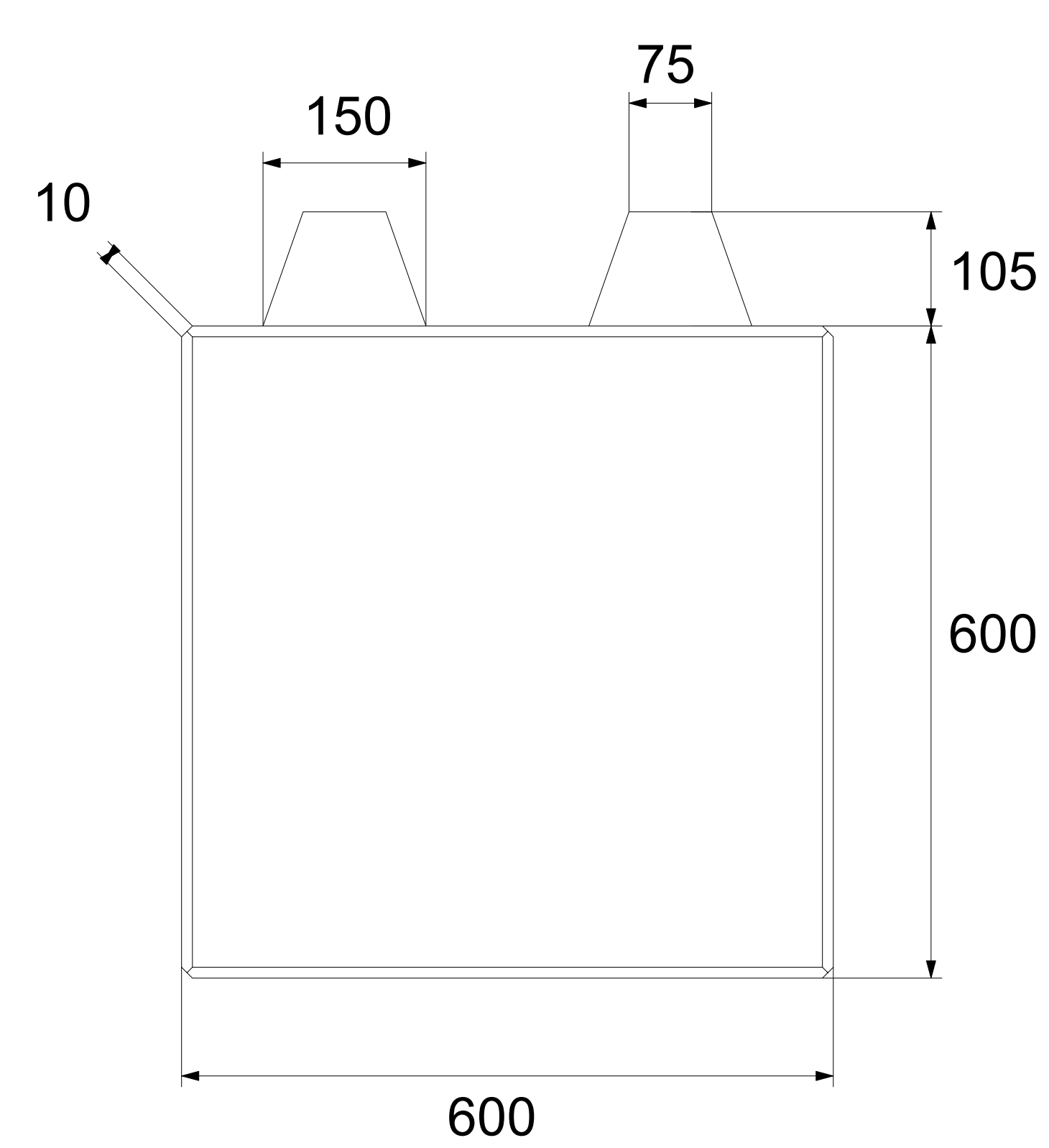
Rzut pionowy
