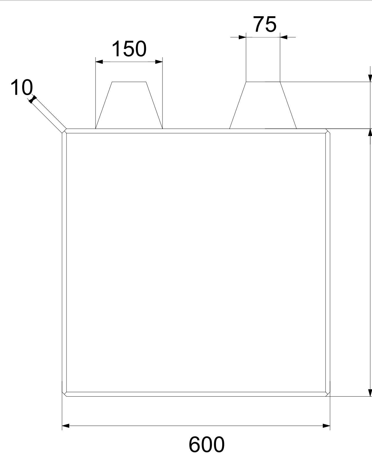
Rzut pionowy
