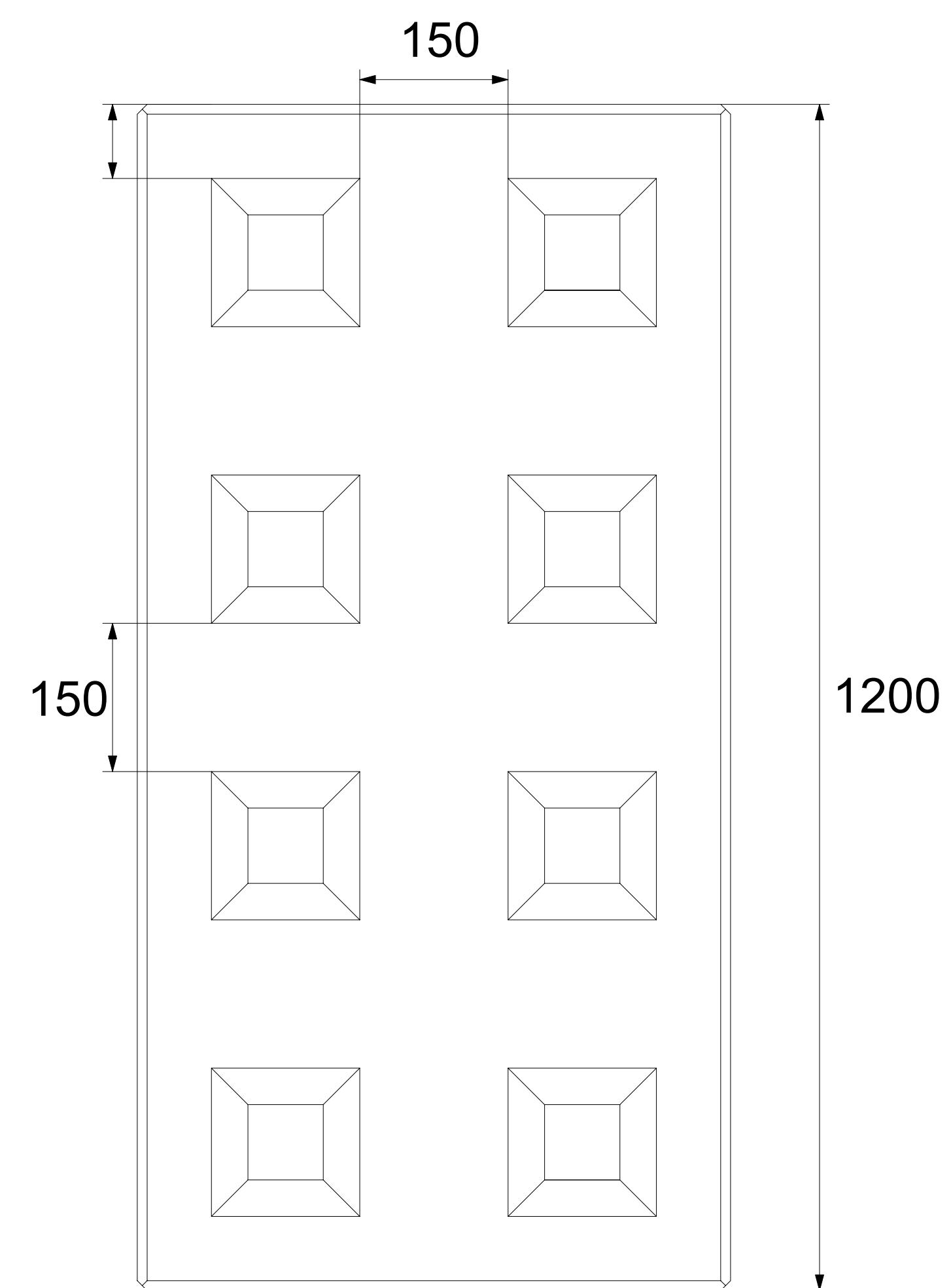
Rzut poziomy
