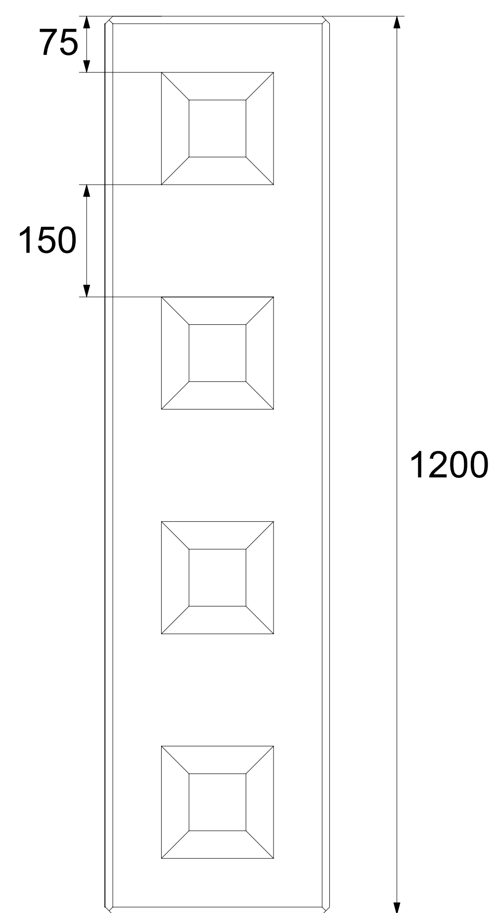
Rzut poziomy
