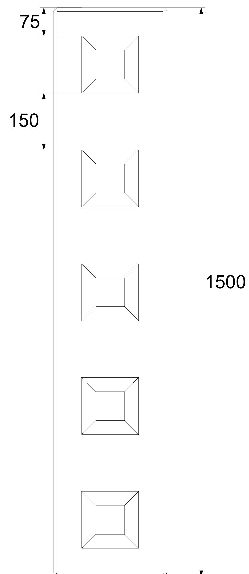
Rzut poziomy
