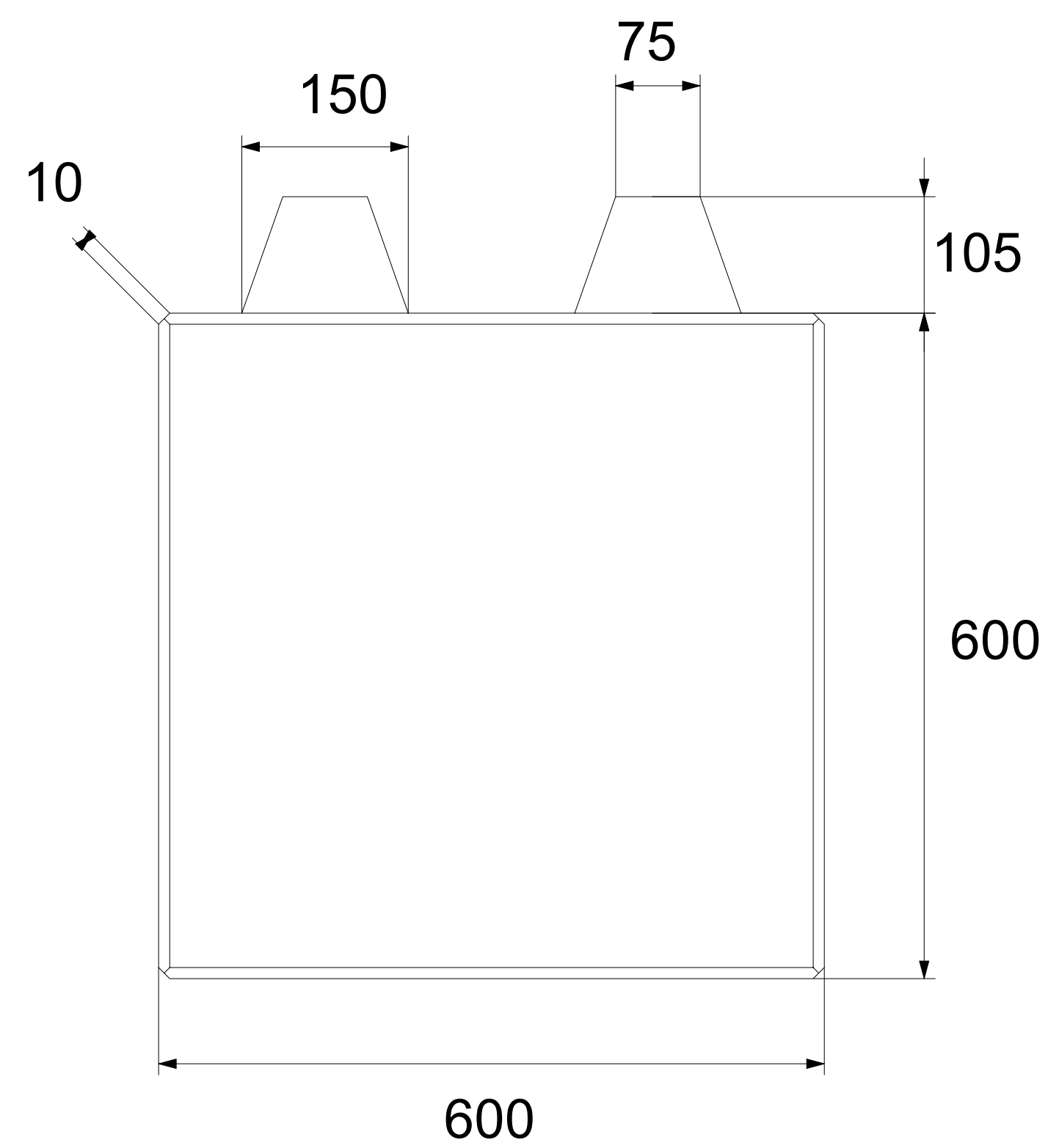
Rzut pionowy
