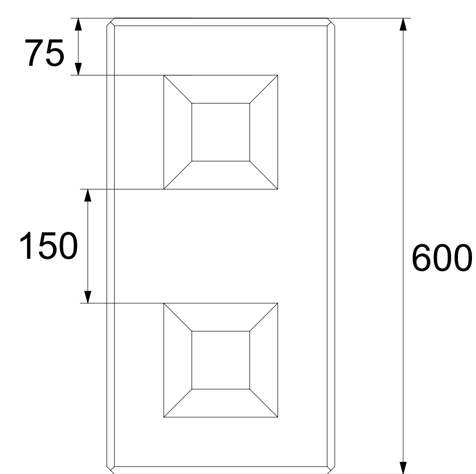
Rzut poziomy
