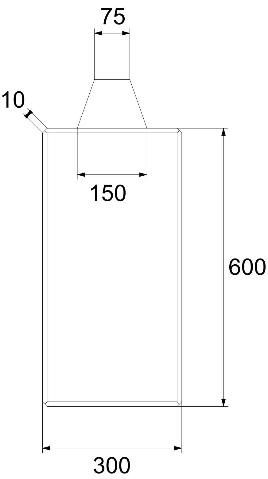
Rzut pionowy
